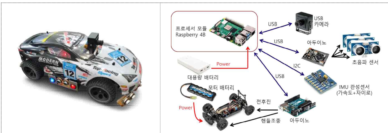
< 자율주행 모형차량 >
